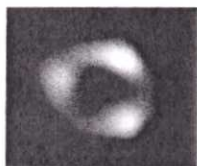
EHT COLLABORATION
