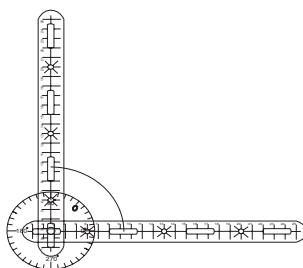
Fig. 4.3: Right angle
