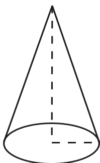
Fig. 12.5 (Cone)
