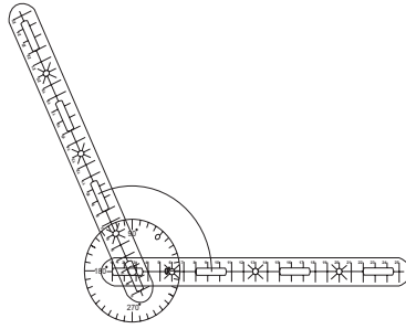
Fig. 4.4: Obtuse angle
