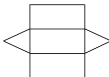
(g) Pyramid
