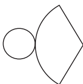
(d) Cone
