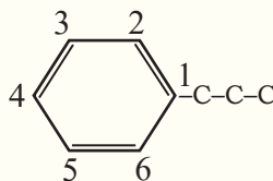
चित्र 5.4 : फेनिल प्रोपेन इकाई
