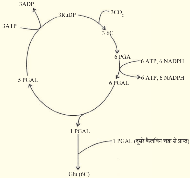
चित्र 2.4 : कैलविन चक्र की रूपरेखा।
