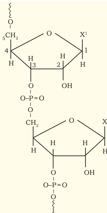
चित्र 4.4 : राइबोन्यूक्लीइक अम्ल (आर.एन.ए.) का एक अंश।
