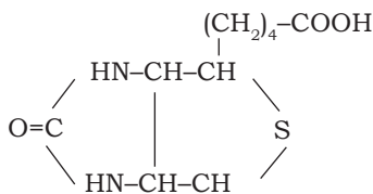
बायोटीन (Biotin)
