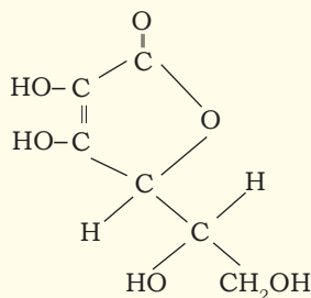
विटामिन सी
