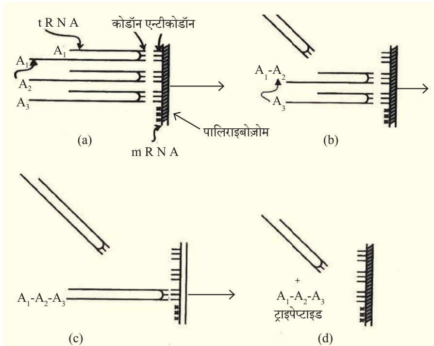
चित्र 4.8 : तीन ऐमीनो अम्लों से निर्मित ट्राइपेप्टाइड का जैव-संश्लेषण (सैद्धांतिक चित्रण)।
