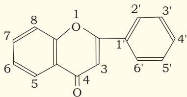
फ्लैवोन (Flavone)
