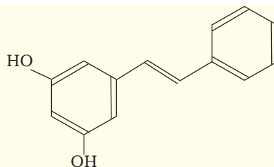
पिनोसिल्विन (Pinosylvin)
