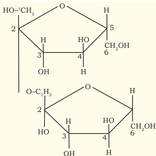
चित्र 3.3 : इनलिन में फ्रक्टोज की दो इकाइयों का पारस्परिक बंध।
