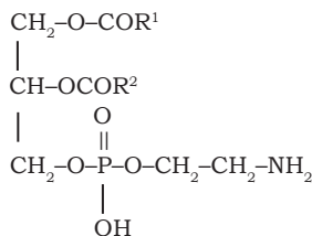
(एक फॉस्फोलिपिड)
