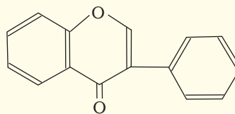
आइसोफ्लैवोन (Isoflavone)
