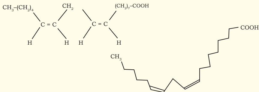
चित्र 6.1 : लिनोलीइक अम्ल
