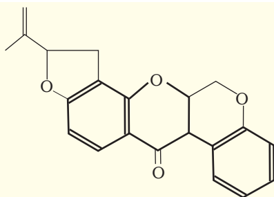
रोटीनोन (Rotenone)
