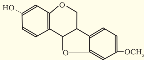
मेडीकार्पिन (medicarpin)
