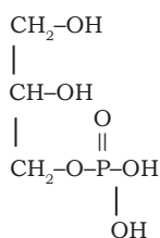
(ग्लिसरोफॉस्फोरिक अम्ल)
