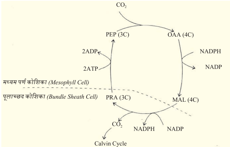
चित्र 2.5 : हैच-स्टैक चक्र की रूपरेखा।
