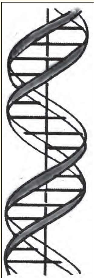
चित्र 4.5 : डी.एन.ए. के द्विकुंडलीय (double helix) का रेखाचित्र।
