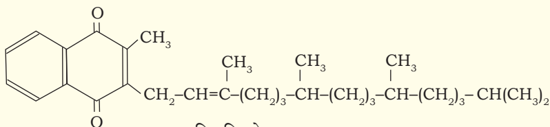
विटामिन के 1 (vitamin K 1 )
