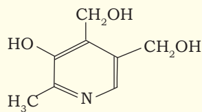
Pyridoxine (II)
