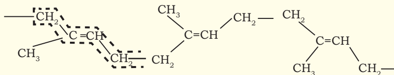
चित्र 5.7 : गटापरचा, बलाटा
