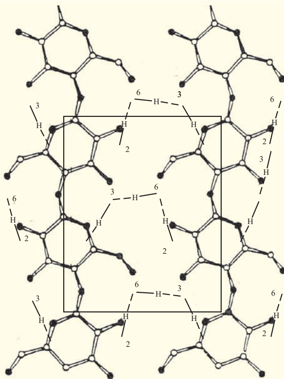
चित्र 3.6 : सेलुलोस में दो पड़ोसी शृंखलाओं के हाइड्रोजन बंध
