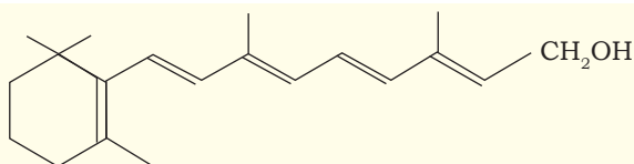
चित्र 6.9 : विटामिन ए
