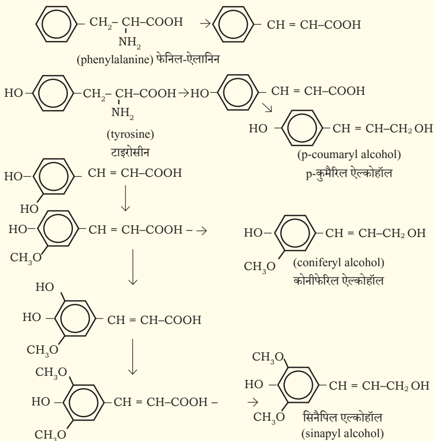
चित्र 5.1 : सिनेमेट पथ (Cinnamate Pathway)
