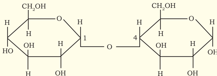
चित्र 3.1 : स्टार्च में ग्लूकोज की दो इकाइयों का पारस्परिक बंध।
